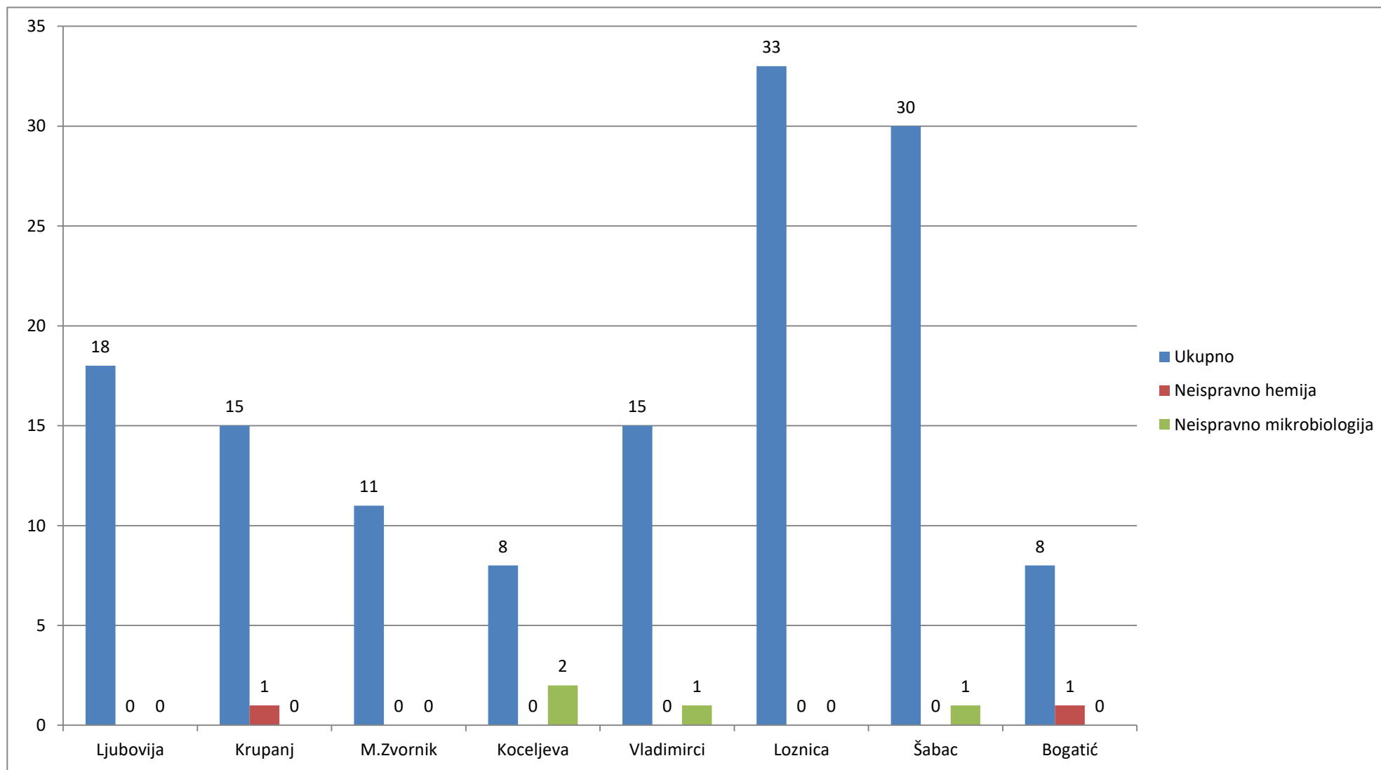
Dijagram ispravnosti vode iz mreže centralnih vodovoda za APRIL 2024 godine.
